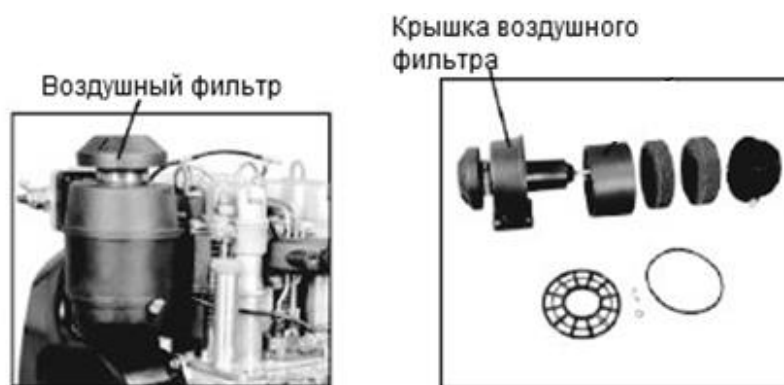
Рисунок 2 – Воздушный фильтр
