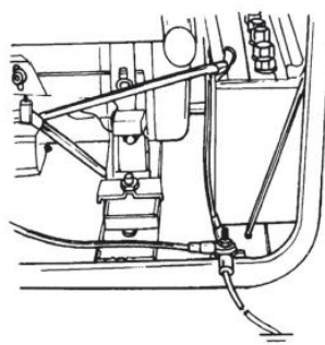
Рисунок 3 – Заземление электроагрегата
